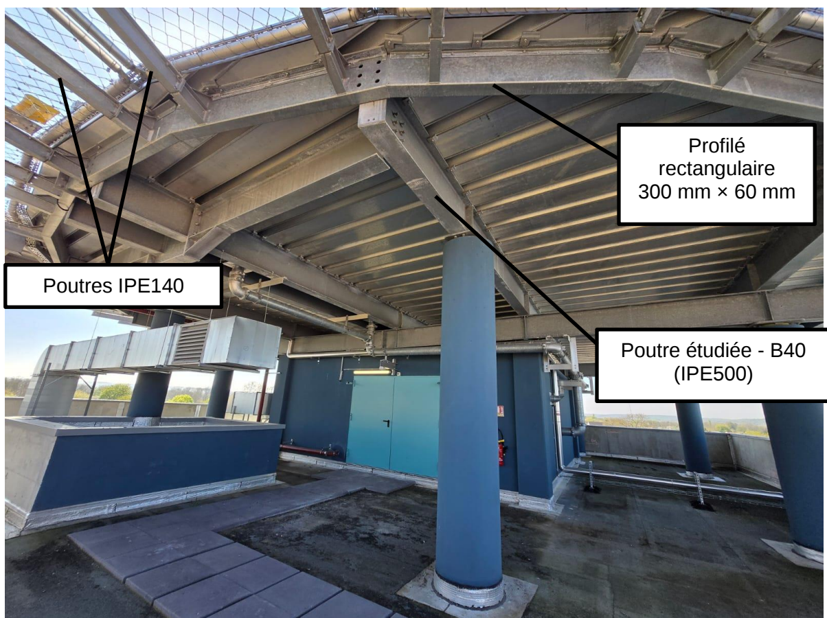
Assemblage des IPE140 avec les profilés Rectangulaire 300 × 60
