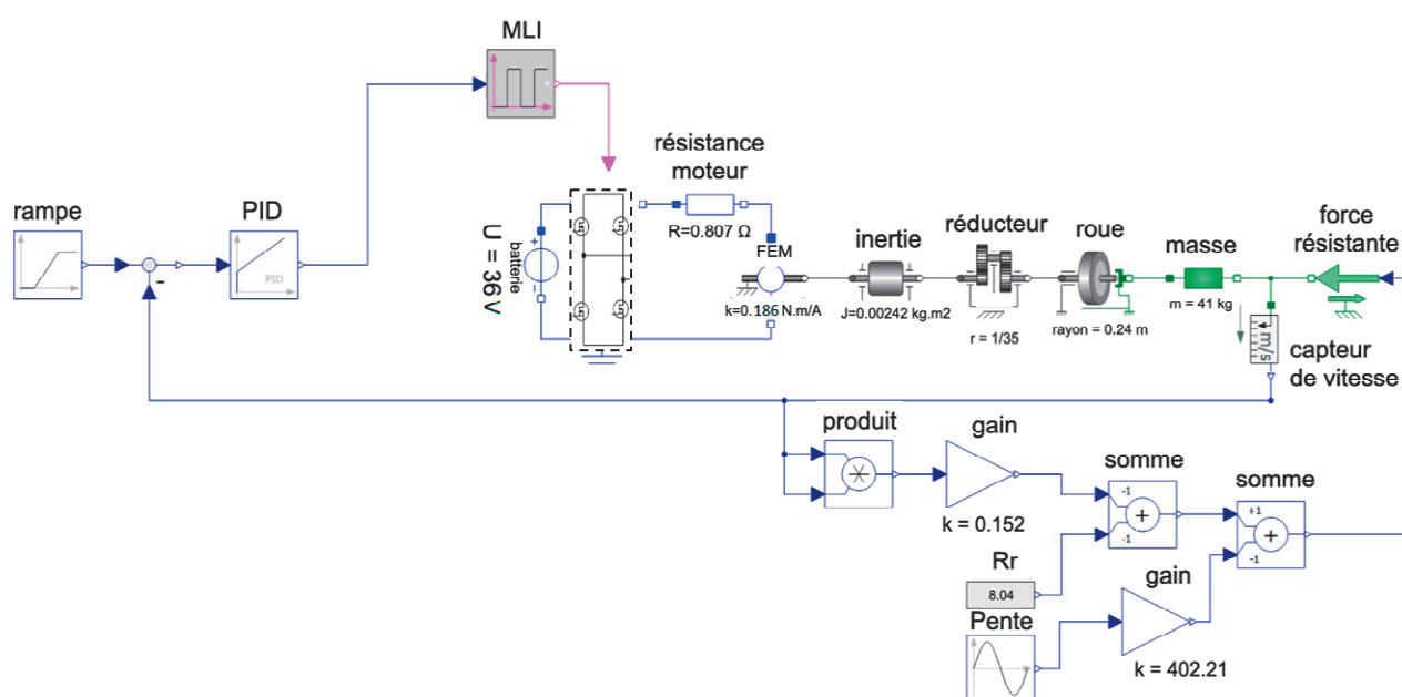
Figure 7 : modèle multi-physique du robot
