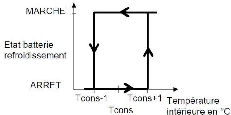
figure 21 : cycle de régulation
