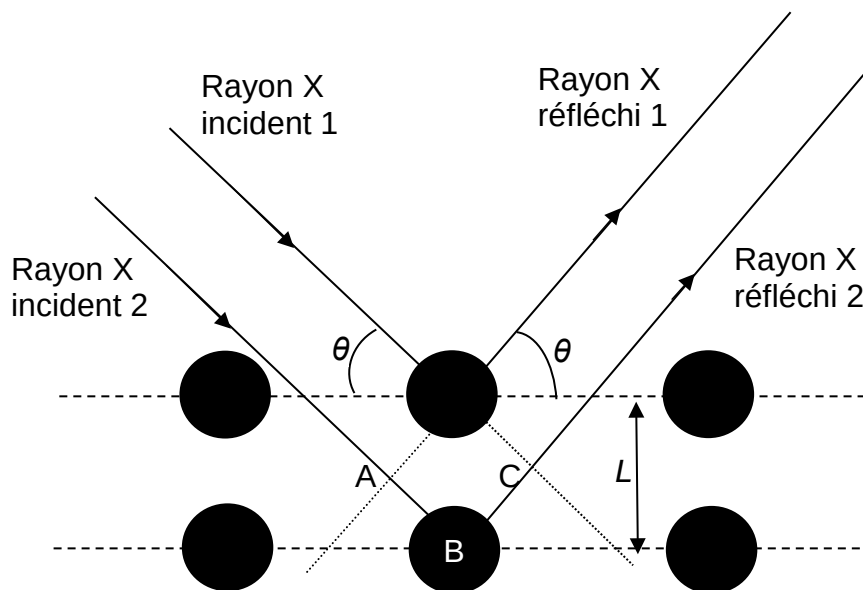
Figure 2. Plan de coupe d'un cristal.
